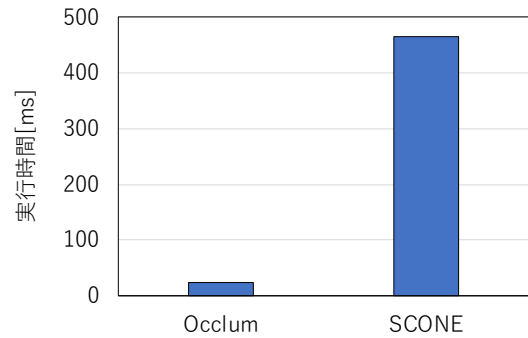
図 16 外部コマンドの呼び出しにかかる時間
