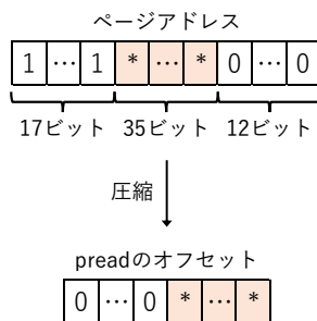
図 6 g_map 関数におけるアドレスの圧縮
