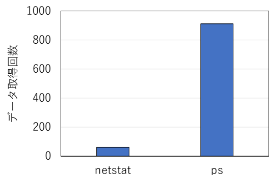
図 13 VM のメモリデータの取得回数
