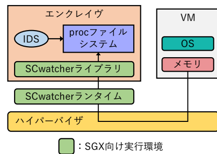
図 3 SCwatcher のシステム構成
