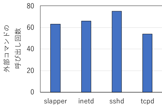
図 15 外部コマンドの呼び出し回数
