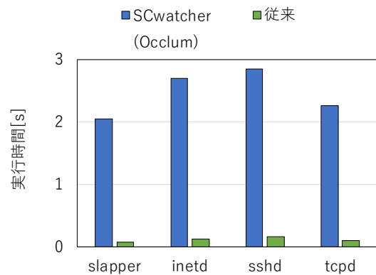
図 17 chkrootkit の実行時間 (従来との比較)
