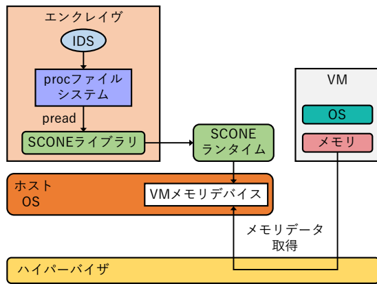
図 5 SCONE を用いた SCwatcher
