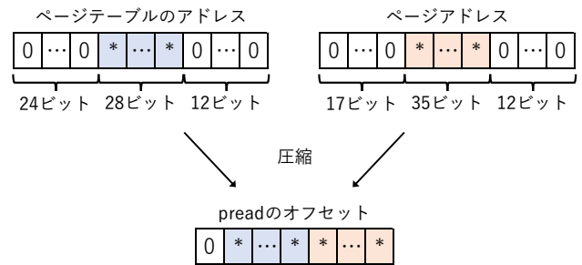
図 7 g_proc_map 関数におけるアドレスの圧縮
