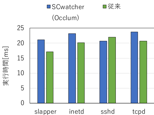
図 19 C 言語版 chkrootkit の実行時間
