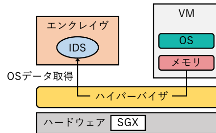
図2 SGmonitor のシステム構成
