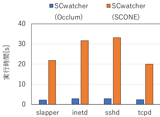
図 14 chkrootkit の実行時間
