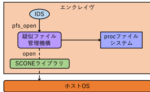
図 8 疑似ファイル管理機構
