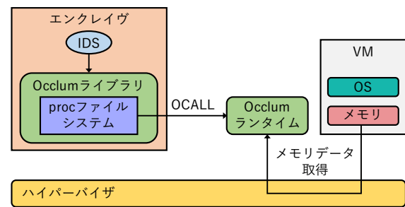
図 4 Occlum を用いた SCwatcher
