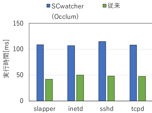
図 18 Python 版 chkrootkit の実行時間
