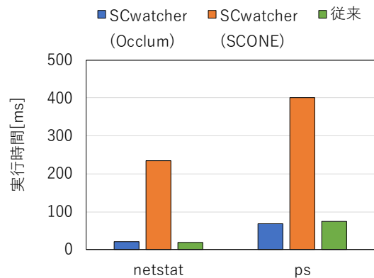
図 12 既存の外部コマンドの実行時間
